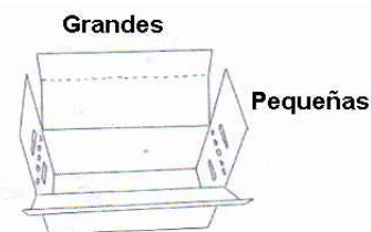
ORDEN DE MONTAJE SUPERIOR (SOLAPAS)
